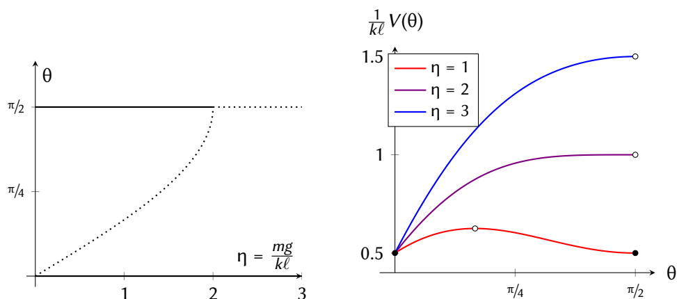
FIGURA 3. (Sinistra) Configurazioni stabili (linea continua) e instabili (linea tratteggiata) al variare del parametro \eta del sistema studiato a pagina 69. (Destra) Energia potenziale V(\theta) per diversi valori di \eta : per ogni curva sono indicati i punti di equilibrio stabile (nero) o instabile (bianco).
