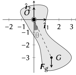
FIGURA 4. Pendolo fisico in moto in un piano verticale.
