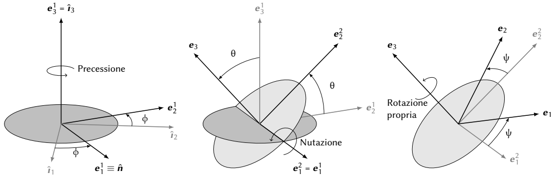
FIGURA 2. Angoli di Eulero.
