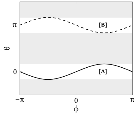
FIGURA 4. Spazio delle configurazioni del sistema biella-manovella. Sono da assumersi condizioni periodiche in entrambi gli assi. La curva continua corrisponde alla relazione tra \theta e \phi in una configurazione di tipo [A], la curva tratteggiata in una configurazione di tipo [B]. Le bande grigie corrispondono a zone proibite.
